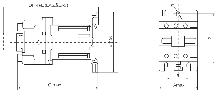
图2 CJX2-40Z~95Z
