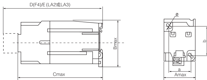
图1 CJX2-09Z~32Z
